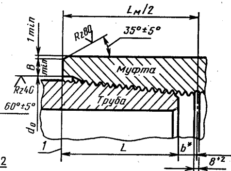
Соединение, свинчивное на станке
