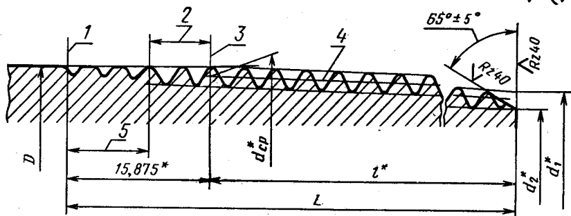
Соединение, свинчивное вручную
