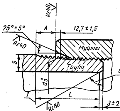
Соединение, свинчивное вручную
